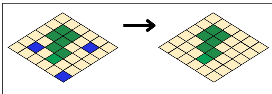
Figura 10. Efecto de la aplicación del filtro espacial.
