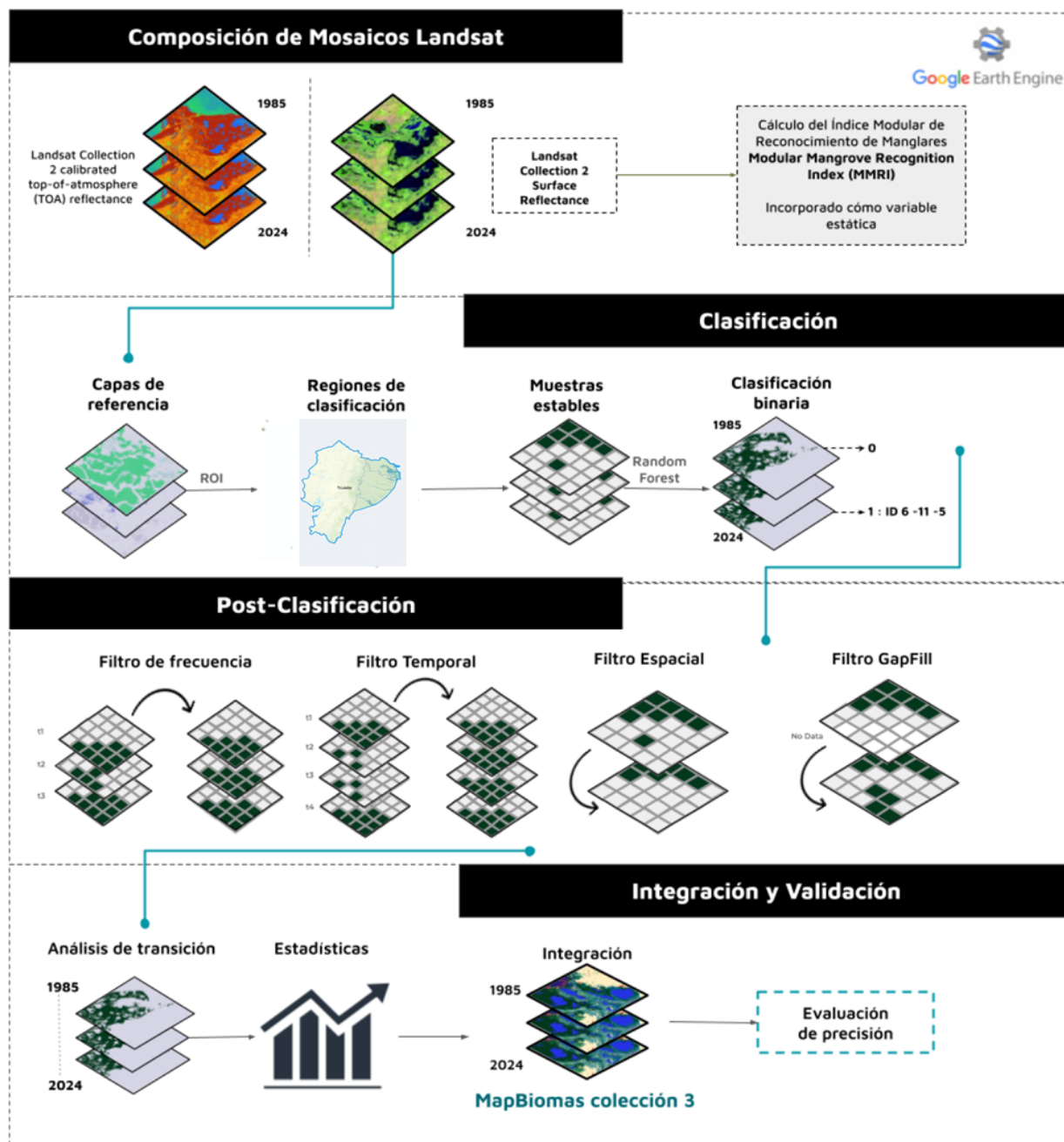
Figura 2. Diagrama metodológico para la identificación de coberturas inundables.
